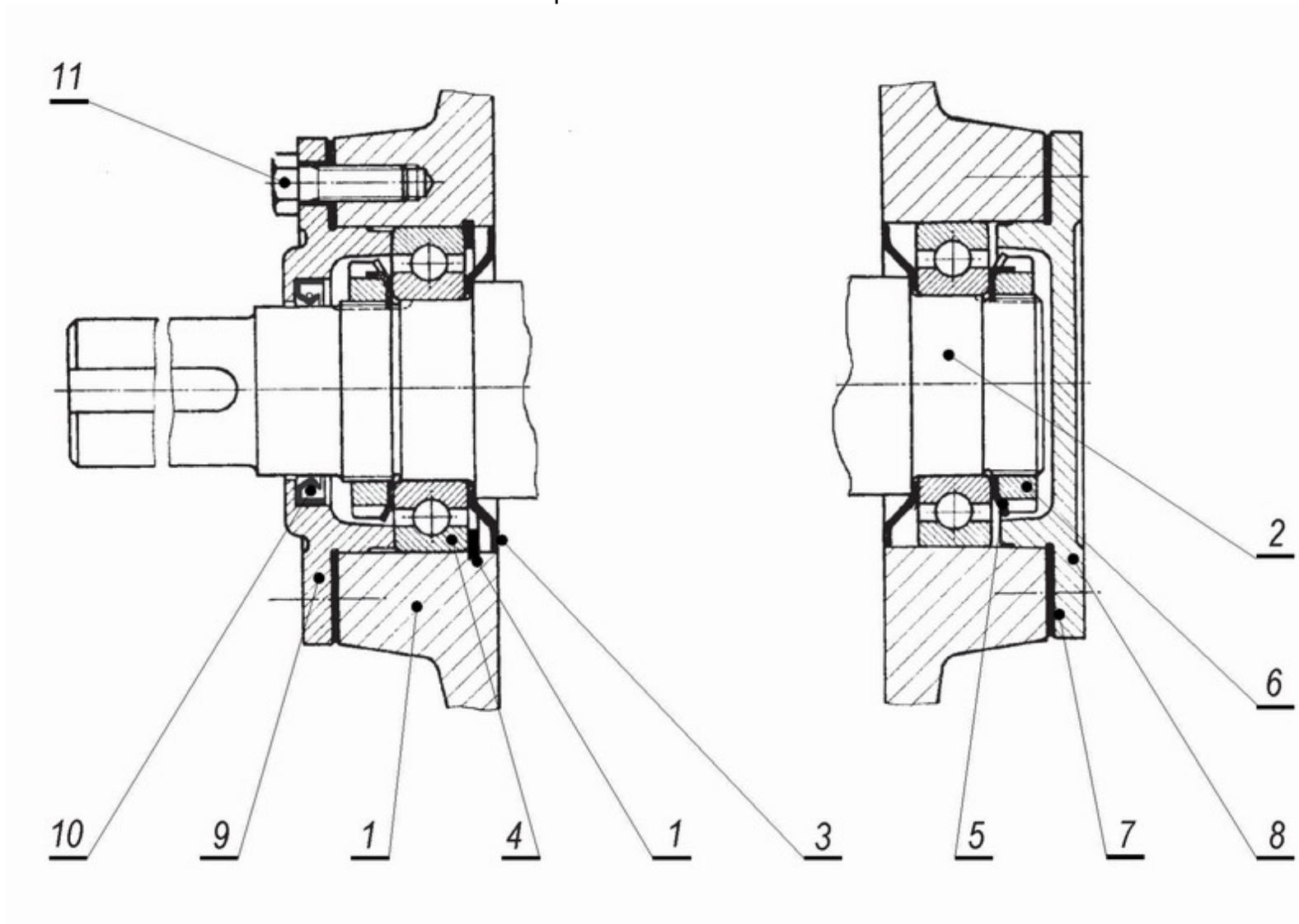
Primer uležištenja vratila
